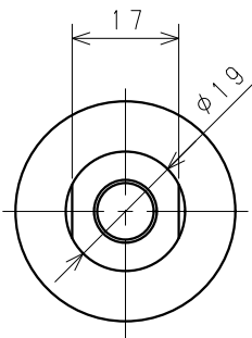
Y-Y' 断面図
